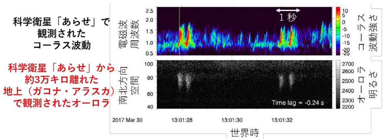
図2. 科学衛星「あらせ」で観測した数百ミリ秒持続期間を示すコーラス波動のパケットと地上(ガコナ・アラスカ)で観測されたオーロラの一対一対応 宇宙で発生したコーラス波動に伴う波動粒子相互作用に関する情報が磁力線を通じて地上からオーロラとして仔細に可視化されている
