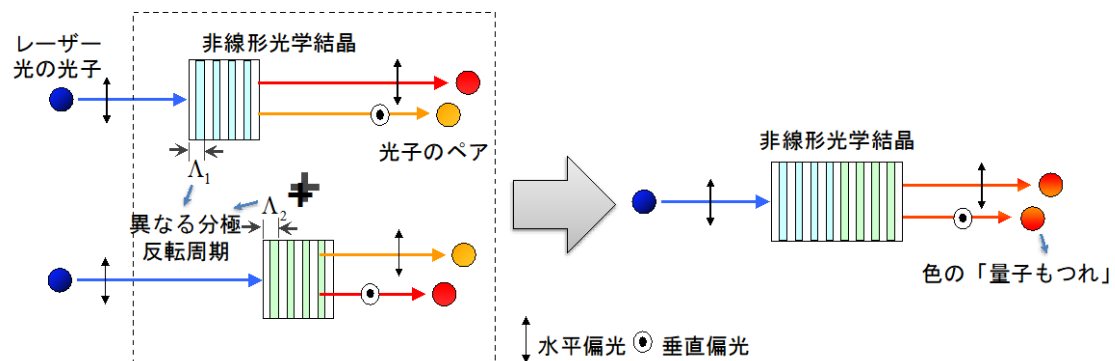
図1:周波数の量子もつれ光子発生方法概念図。レーザー光子は非線形光学結晶内で光子のペアに分裂し得るが、2つの異なる領域で発生しうる光子の周波数と偏光の状態が互い違いになっている相関を持っており、光子のペアは量子もつれ状態となる。従来の方法で必要であった干渉計等の複雑な光学系や損失の大きい光フィルターを必要とせず、簡便に周波数の量子もつれが発生可能となった。
