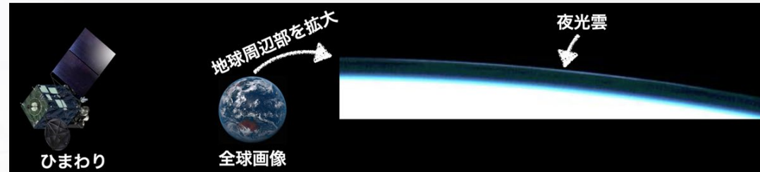
図: 静止軌道衛星ひまわりによる夜光雲の観測
